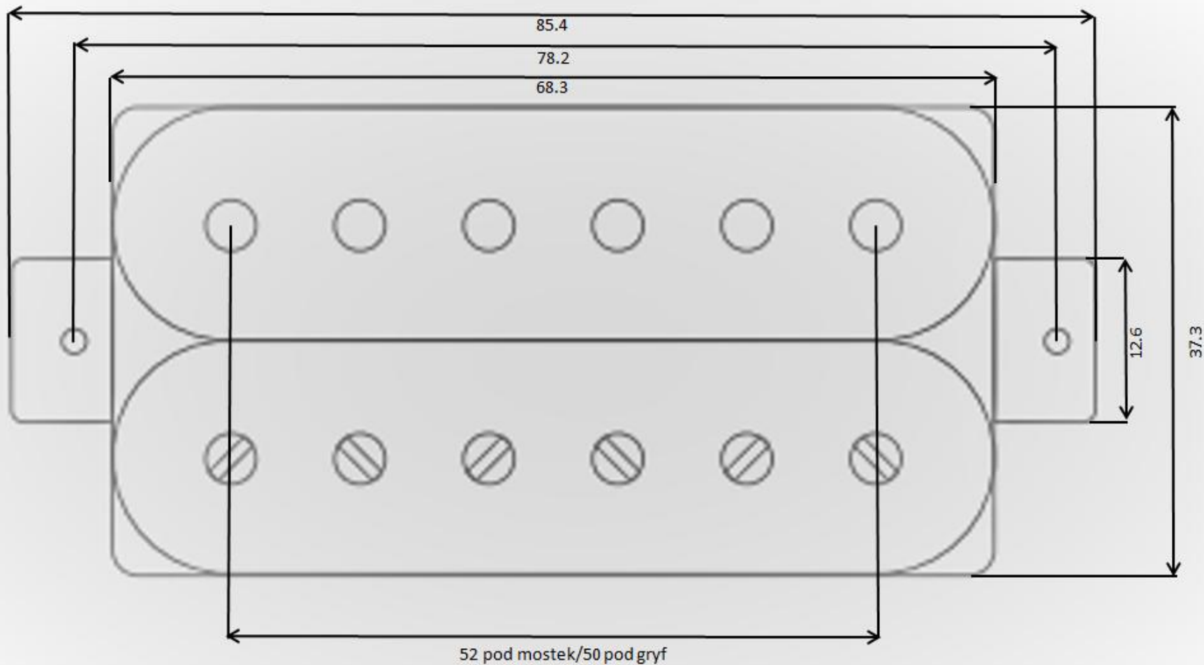
Humbucker - wszystkie wymiary podane są w milimetrach. Wysokość przetwornika 21.8mm
