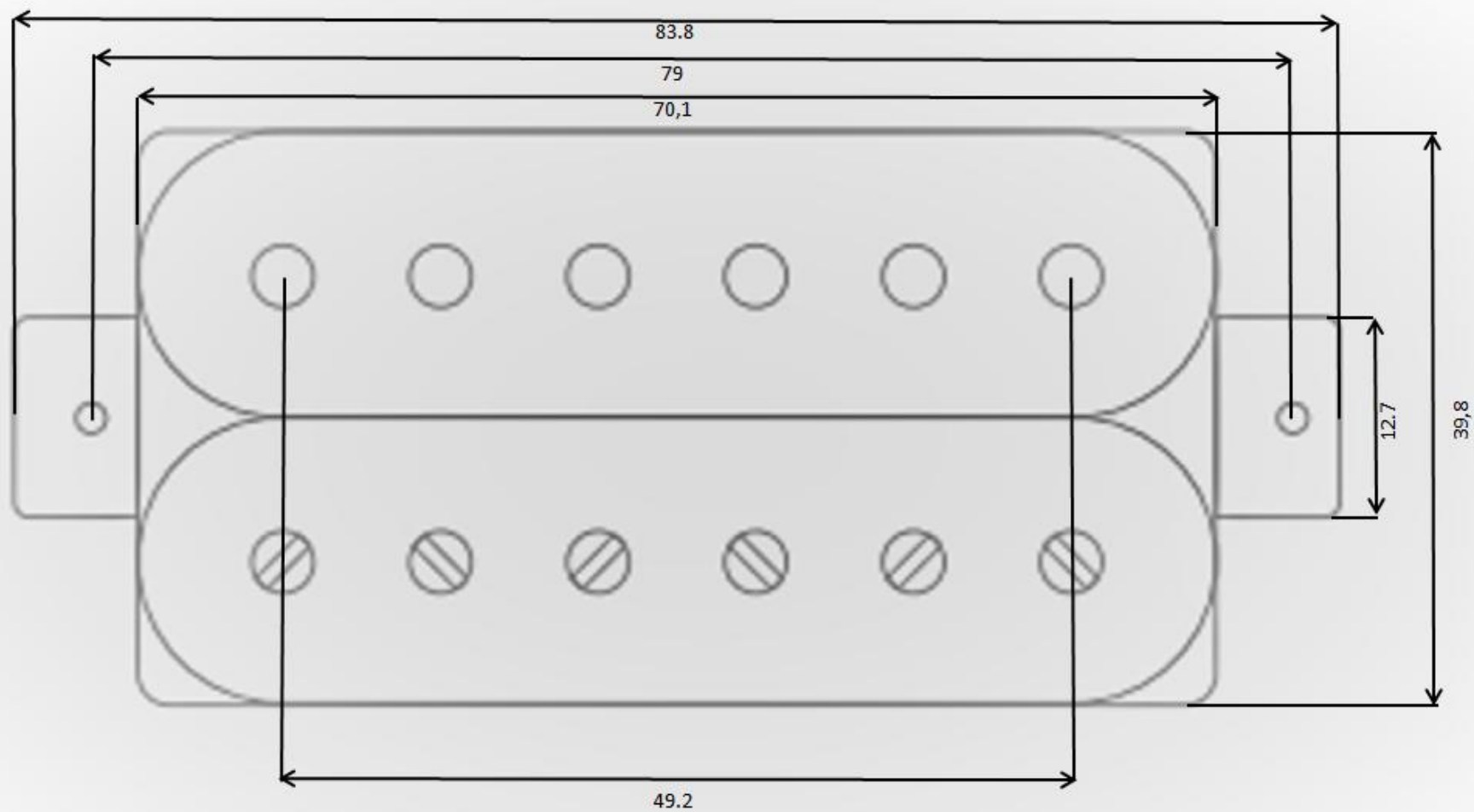
Humbucker Signature - wszystkie wymiary podane są w milimetrach. Wysokość przetwornika 28mm
