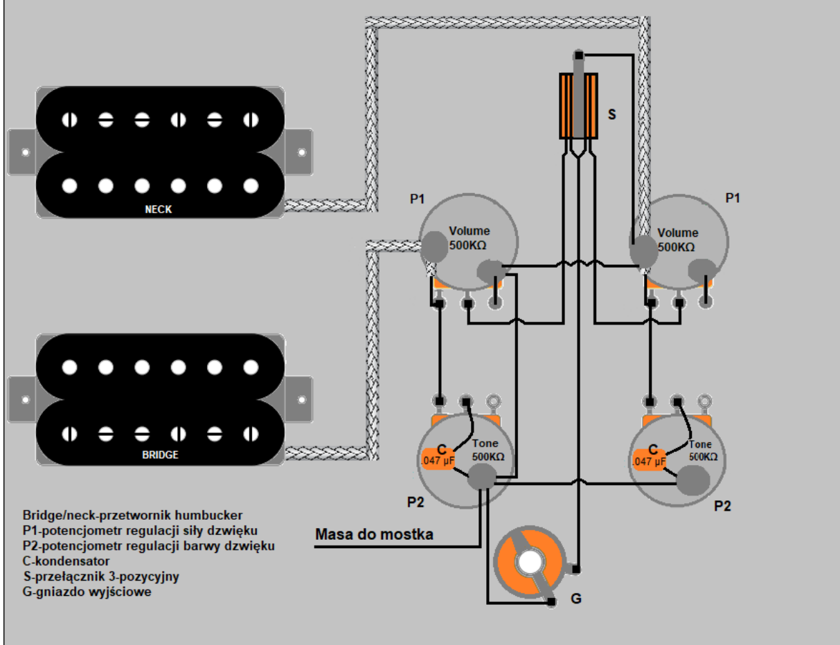
Schemat połączeń przetworników typu humbucker w gitarze elektrycznej (przewód 1-żyłowy)
