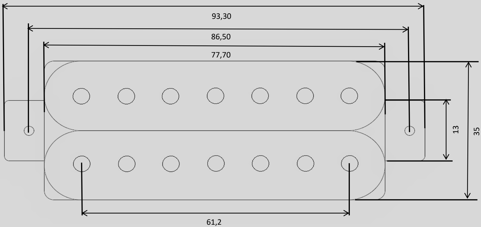
Humbucker 7 - string J&J Artin - wszystkie wymiary podane są w milimetrach. Wysokość przetwornika z nabiegunnikami 20,6 mm.
